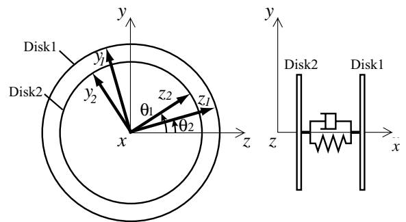
Fig. 7 Motor element.
