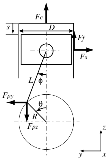
Fig. 4 Piston-conrod element.
