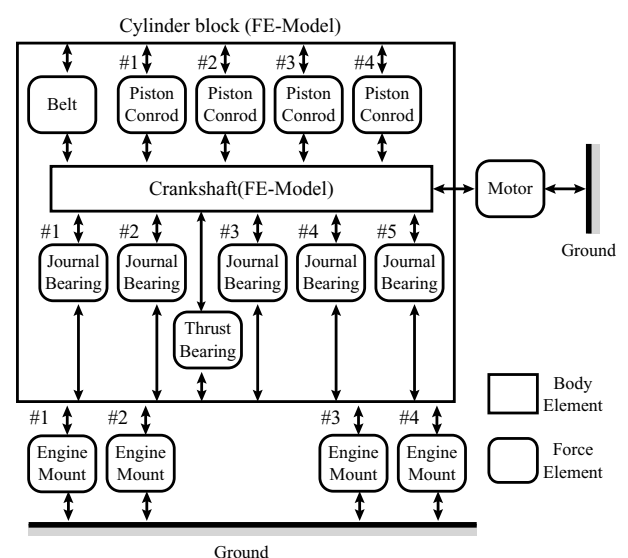
Fig. 1 Schematic of EVAS.
